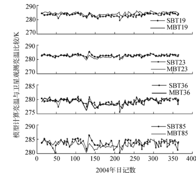
图 4 模型计算区域 B 10—85GHz 亮温与 SSM/I 实际观测亮温的比较(SBT:SSM/I 观测亮温, MBT:模型计算亮温)
