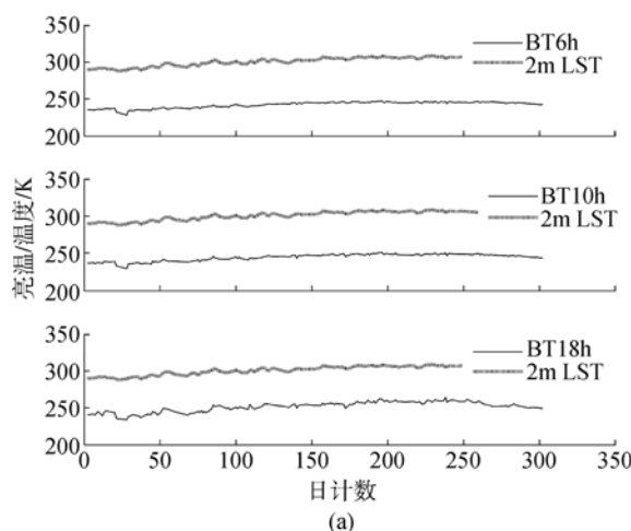
图 5 AMSR-E 6-18GHz 极化亮温和 2m 地温的日变化趋势
